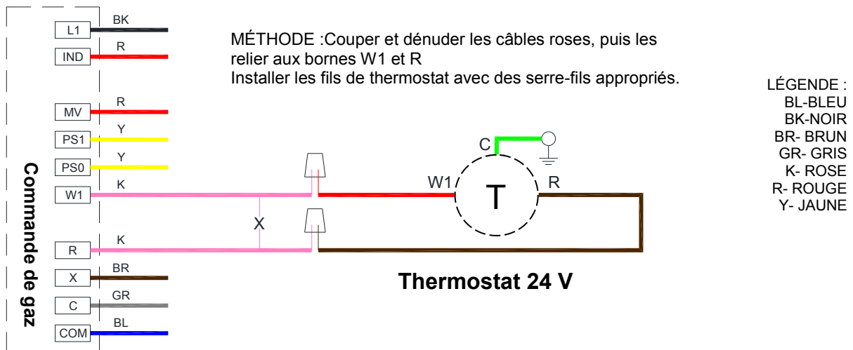
Figure 5c. Installation de plusieurs radiateurs, commande 24 V
