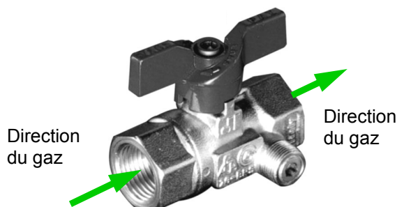
Figure 3. Orientation correcte de la vanne à boisseau
