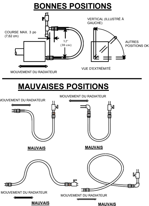
Figure 4. Installation correcte du raccord de gaz flexible
