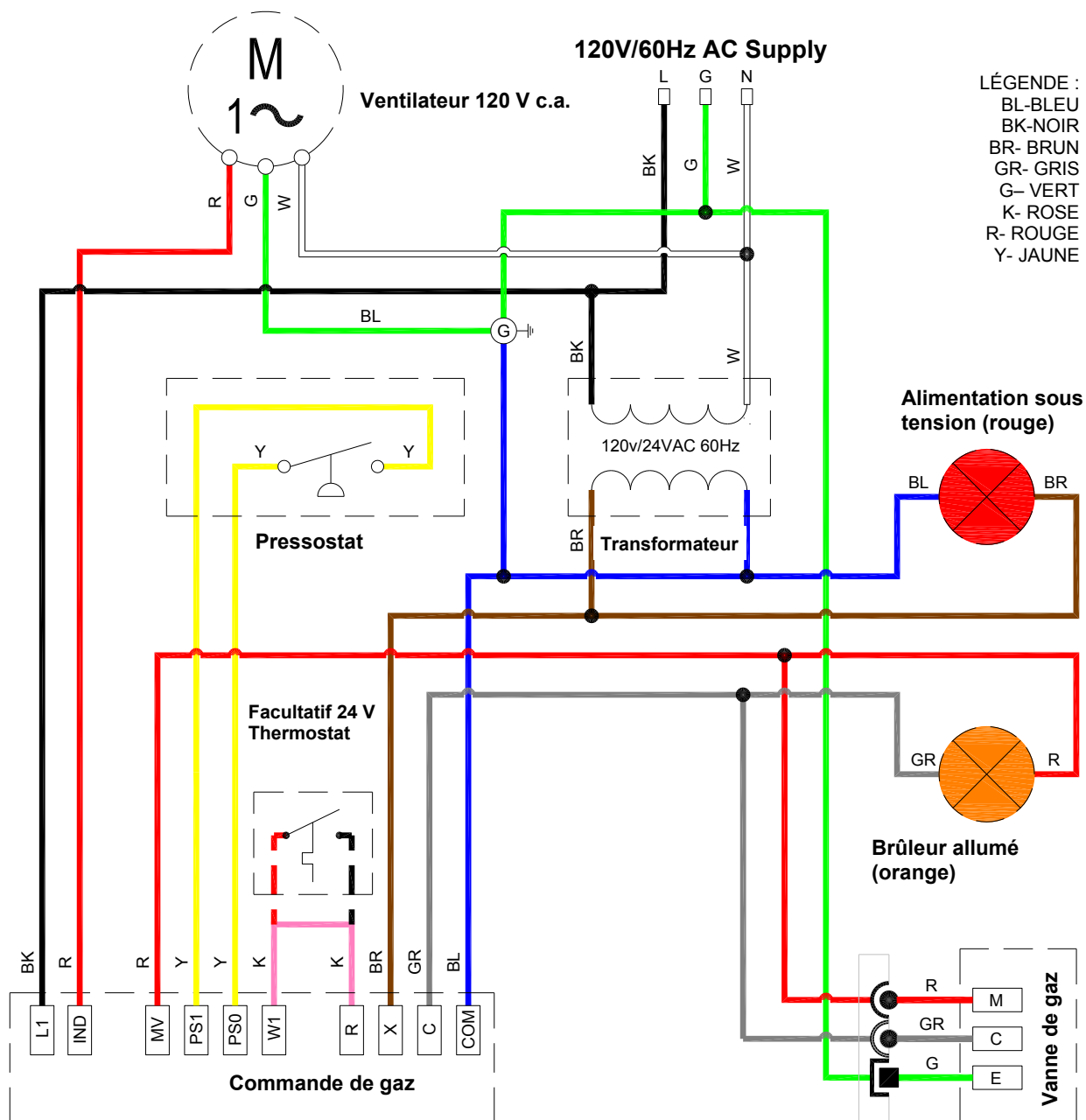
Figure 6. Diagramme électrique du brûleur interne
