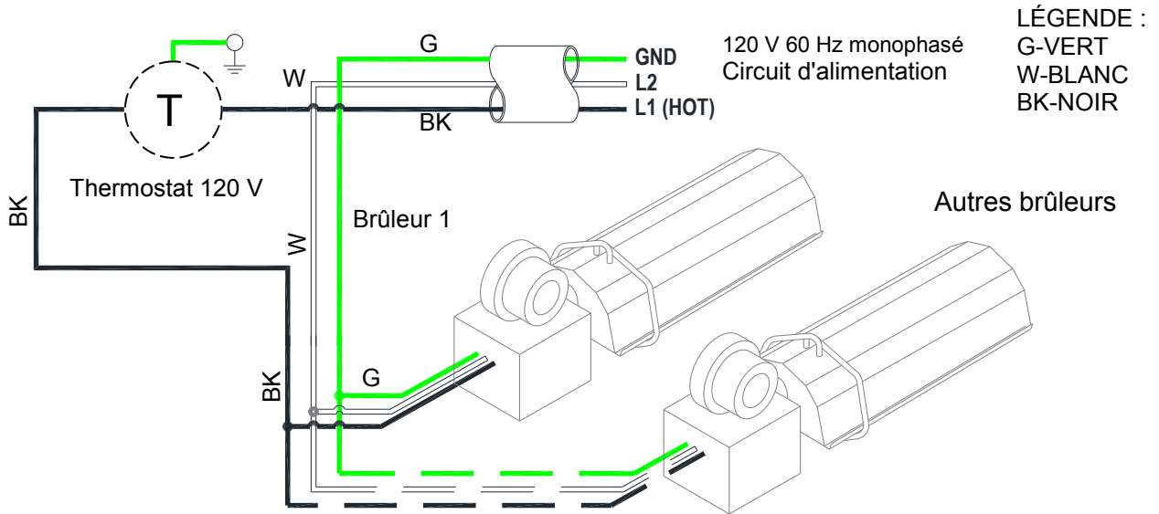
Figure 5a. Installation d'un ou plusieurs radiateurs, commande sous 120 V
