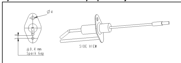
Rys. 10a : Montaż elektrody zapłonowej
