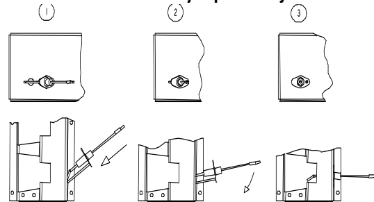
Rys. 10b : Montaż elektrody zapłonowej
