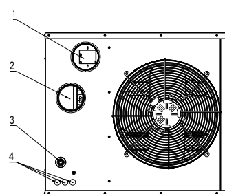
Rysunek 2a: Gniazda powietrza do spalania i układu
