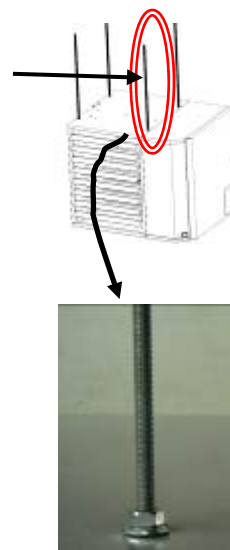
Rysunek 3 Szczegóły podwieszenia
