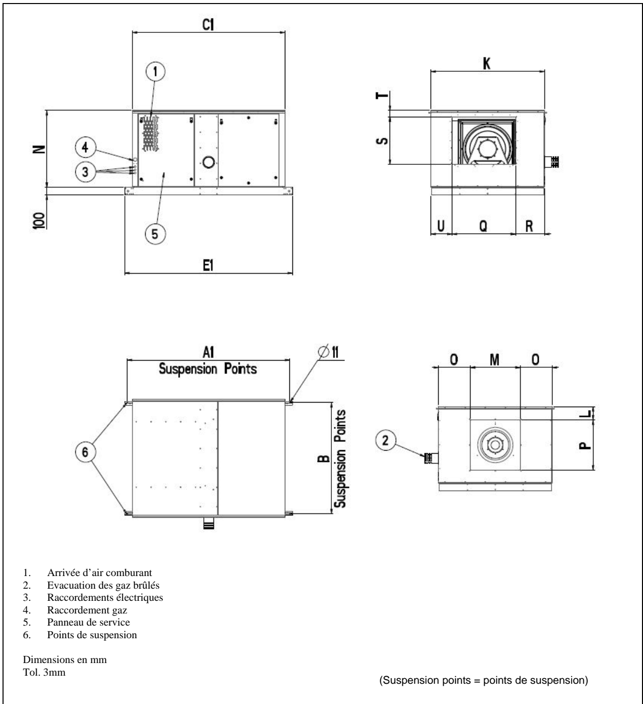
Figure 2.3 : RDH EC sans caisson de filtration
