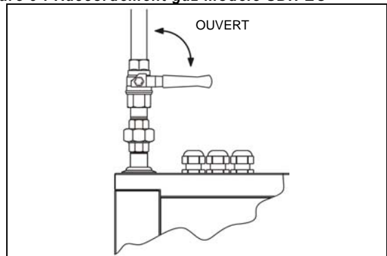
Figure 9 : Raccordement gaz modèle SDH EC
