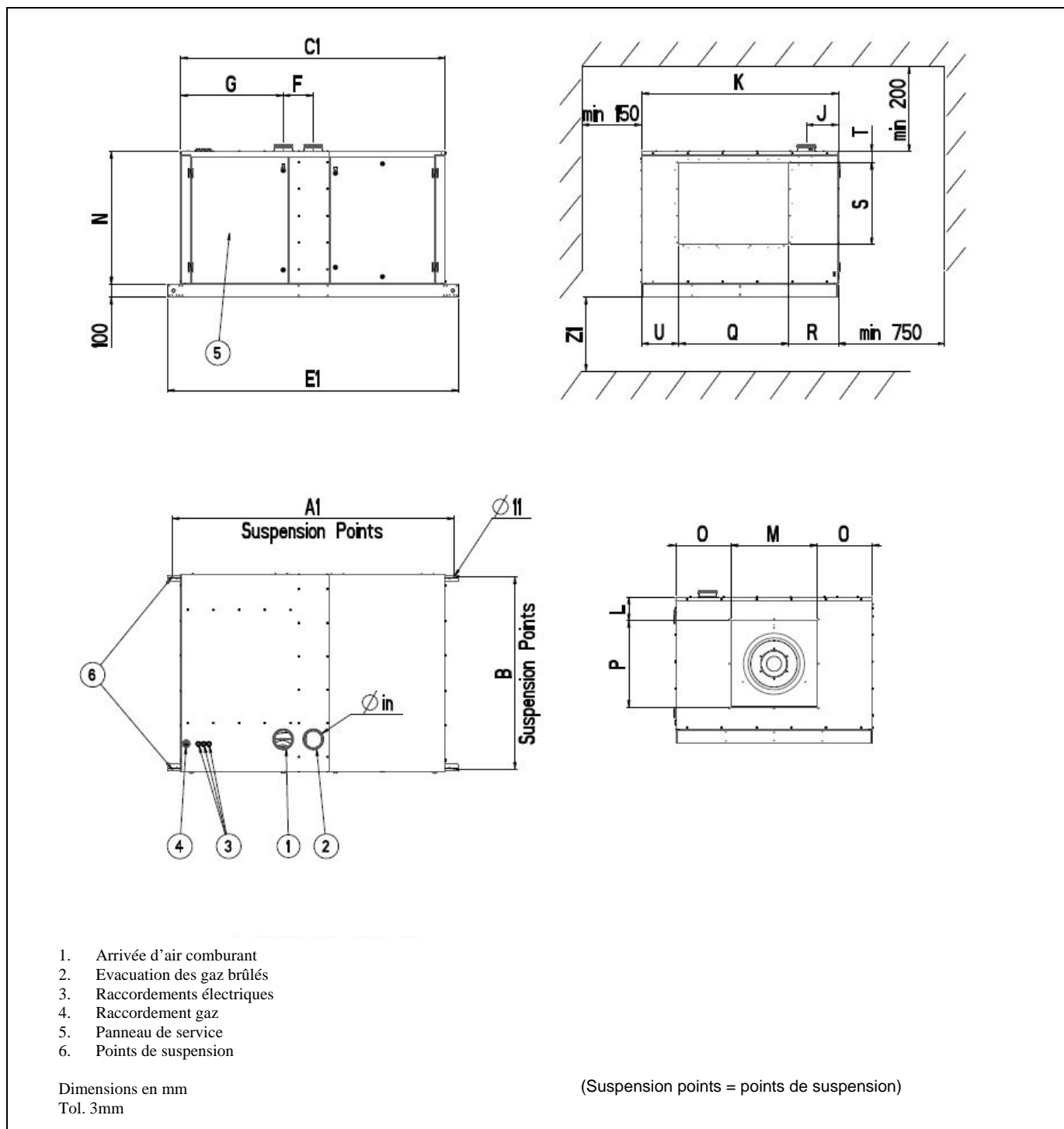
Figure 2.1 : SDH EC sans caisson de filtration
