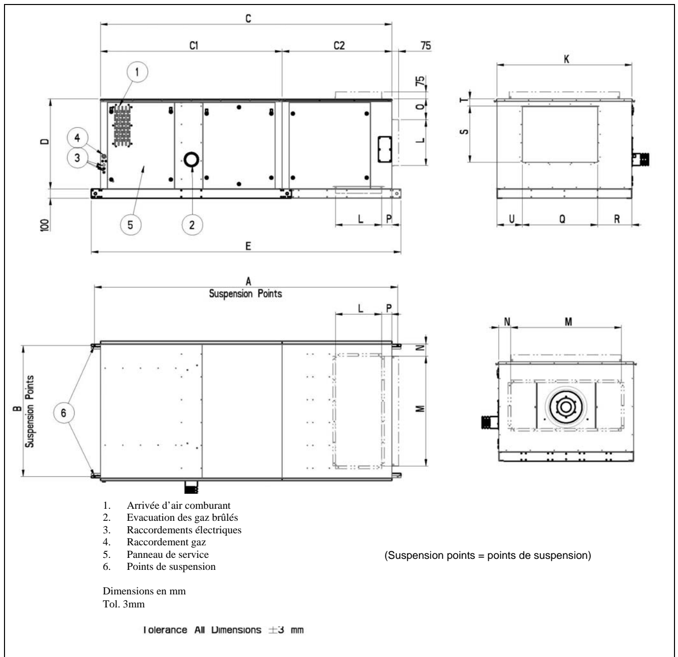
Figure 2.4 : RDH EC avec caisson de filtration
