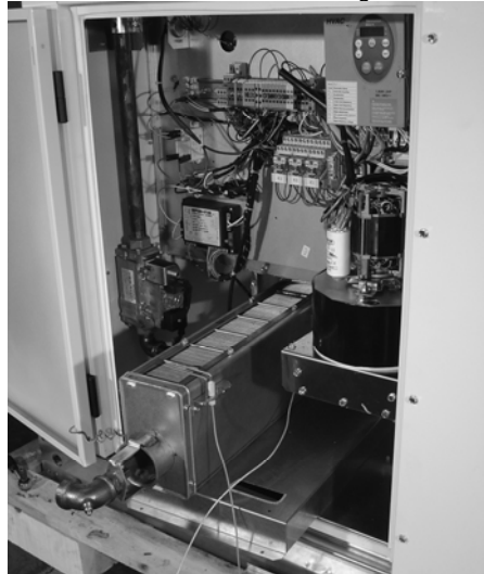
Figure 24 Enlever le corps du brûleur, la sonde de flamme et l'électrode d'allumage
