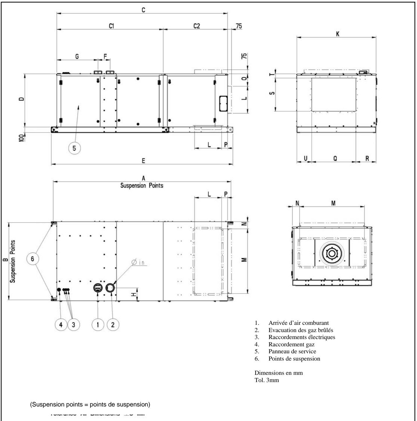
Figure 2.2 : SDH EC avec caisson de filtration
