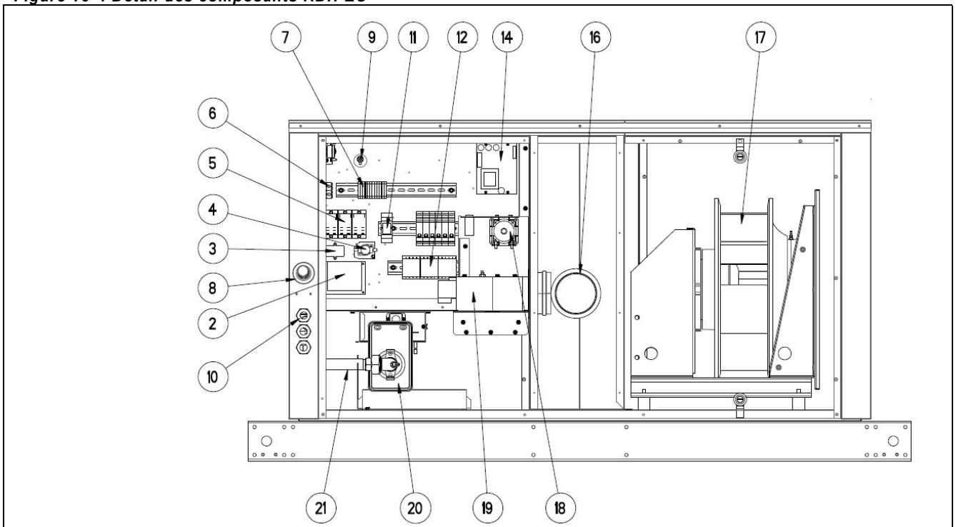
Figure 16 : Détail des composants RDH EC
