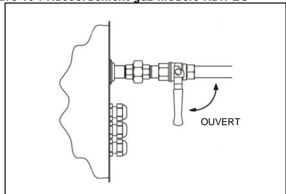
Figure 10 : Raccordement gaz modèle RDH EC
