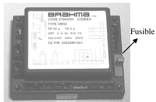
Figure 29 :Relais d'allumage
