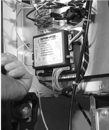
Figure 23 Déconnecter câble de la sonde de flamme sur le relais de flamme
