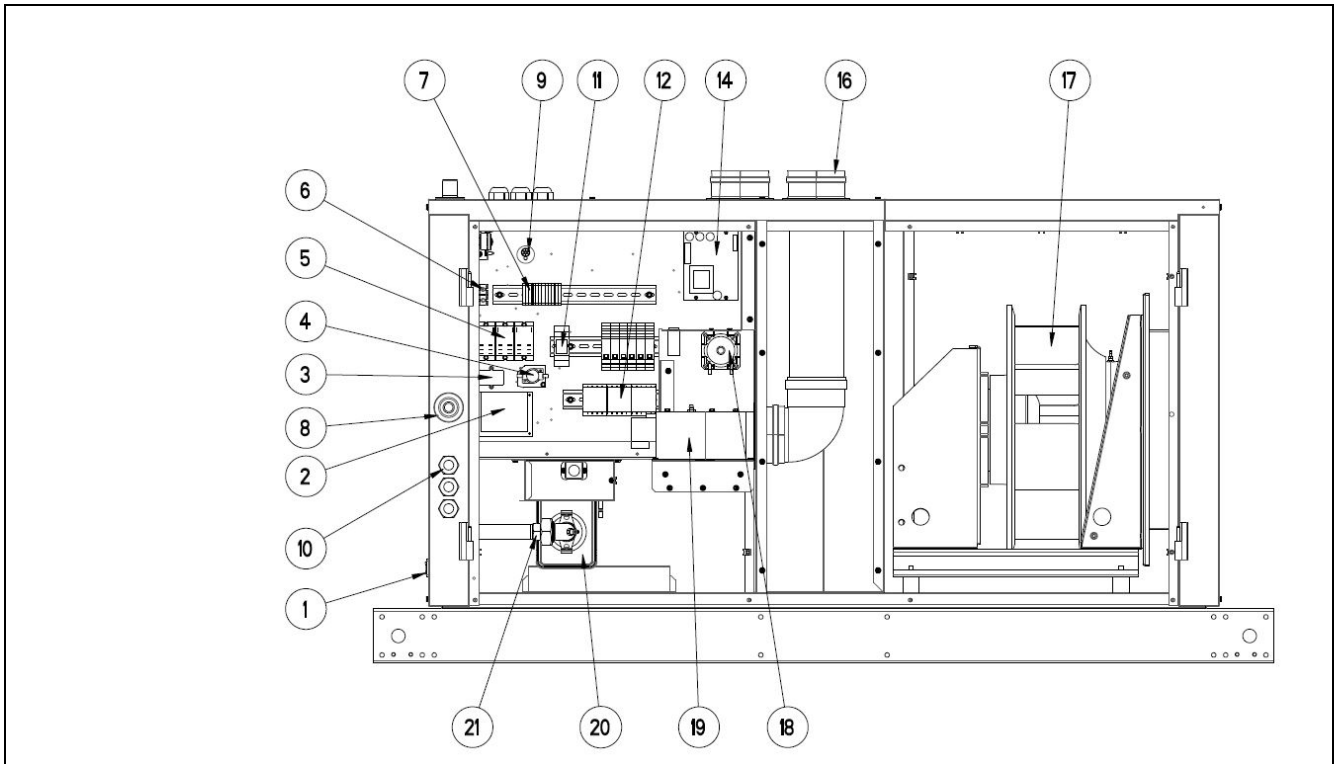
Figure 15 : Détail des composants SDH EC
