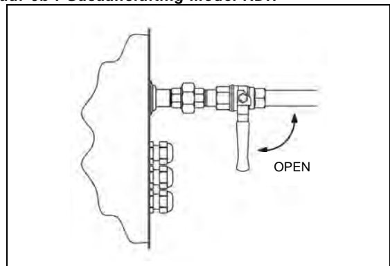
Figuur 9b : Gasaansluiting model RDH
