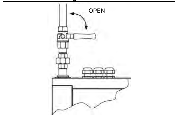
Figuur 9a Gasaansluiting model SDH
