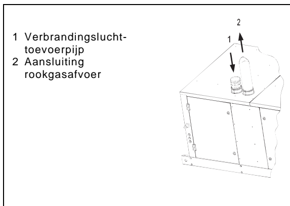
Figuur 6b : Type B installatie Aansluitingen luchttoevoer & rookgasafvoer
