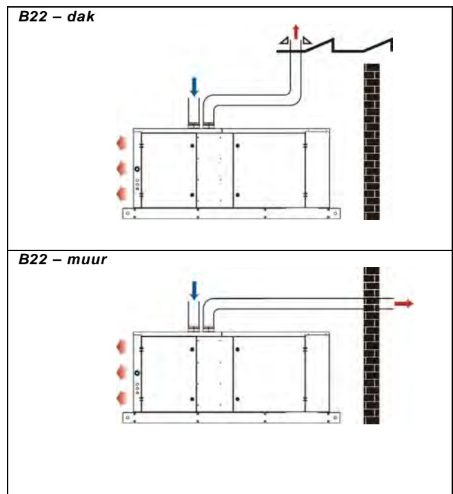
Figuur 6a : Gekeurde schoorsteenuitvoering - type B
