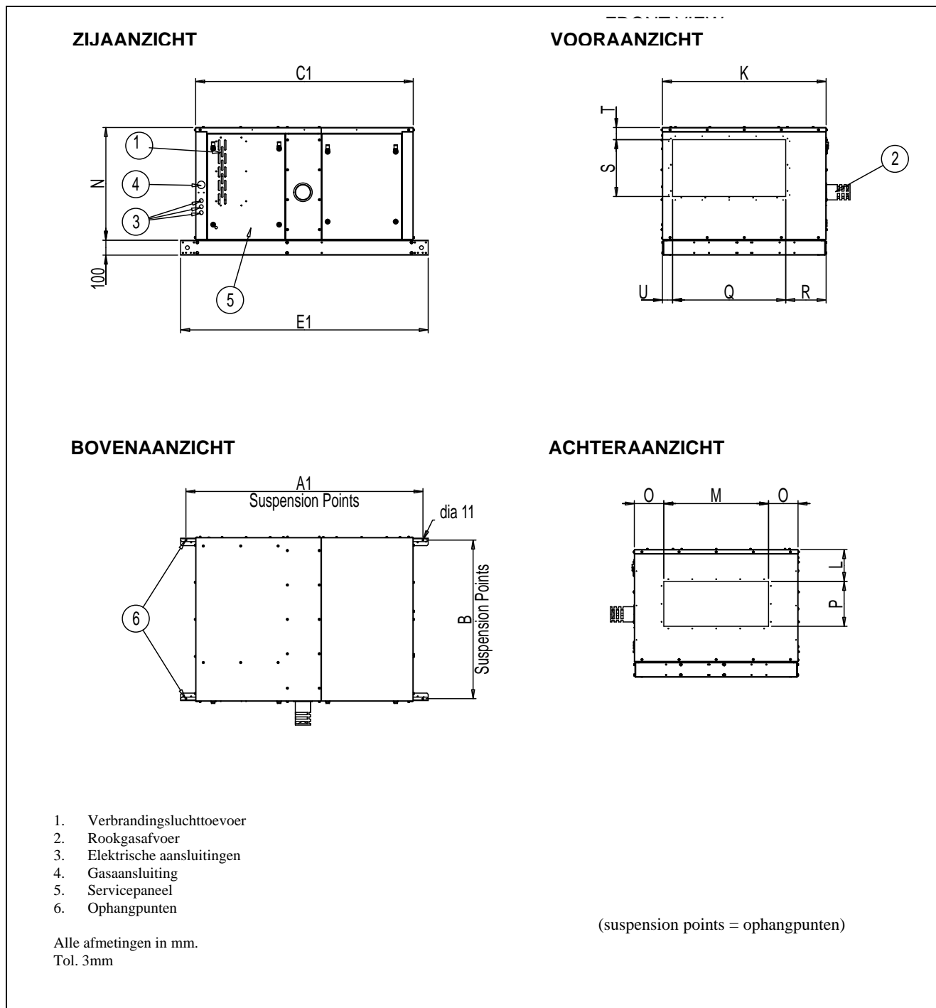
Figuur 2.3 : RDH model- Standaard uitvoering
