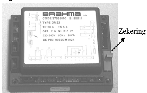
Figuur 29 :Branderautomaat
