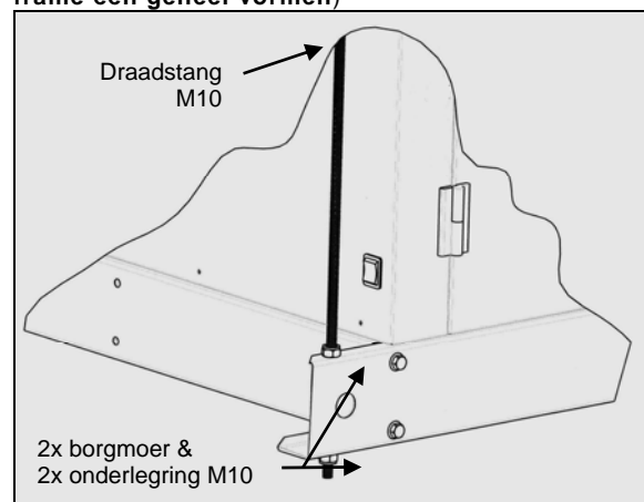
Figuur 3 : Detail bevestiging (enkel indien toestel en frame één geheel vormen)
