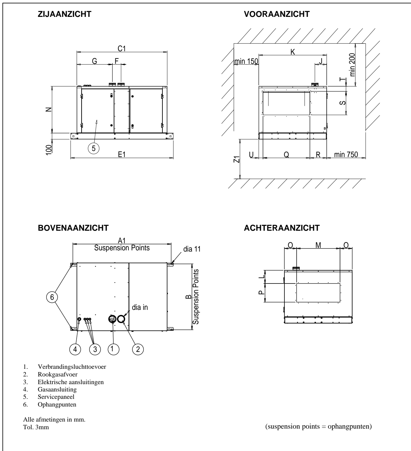
Figuur 2.1 : SDH model – Standaard uitvoering
