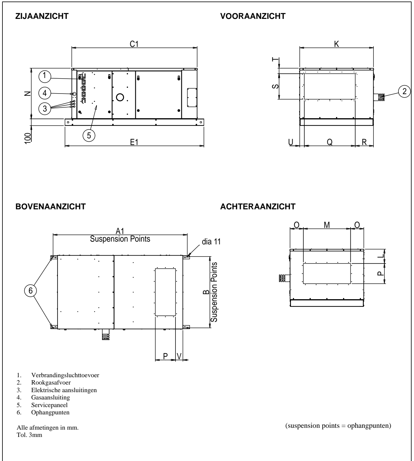
Figuur 2.4 : RDH model-met geïntegreerde filterkast
