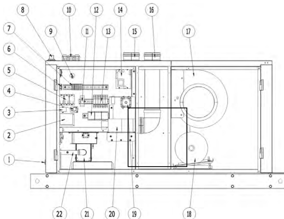
Figuur 16 : Componenten
