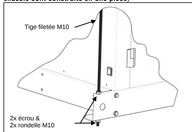
Figure 3 : Détail fixation (seulement si l'appareil et le châssis sont construits en une pièce)
