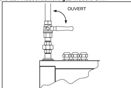
Figure 9a : Raccordement gaz modèle SHH
