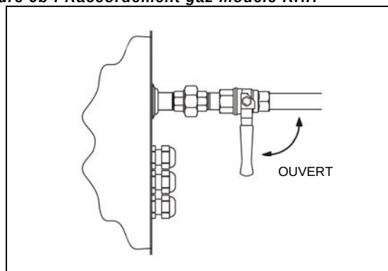
Figure 9b : Raccordement gaz modèle RHH
