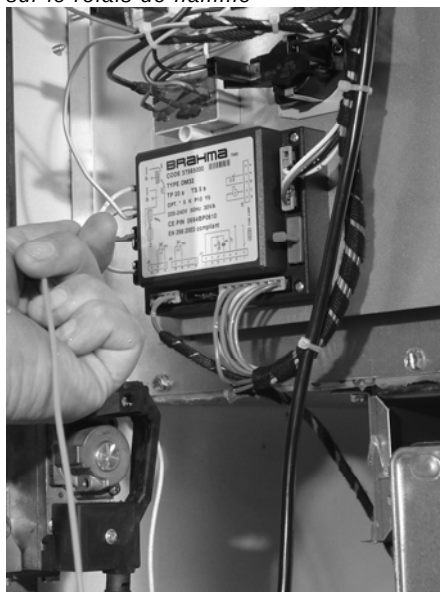
Figure 22 Déconnecter câble de l'électrode d'allumage sur le relais de flamme
