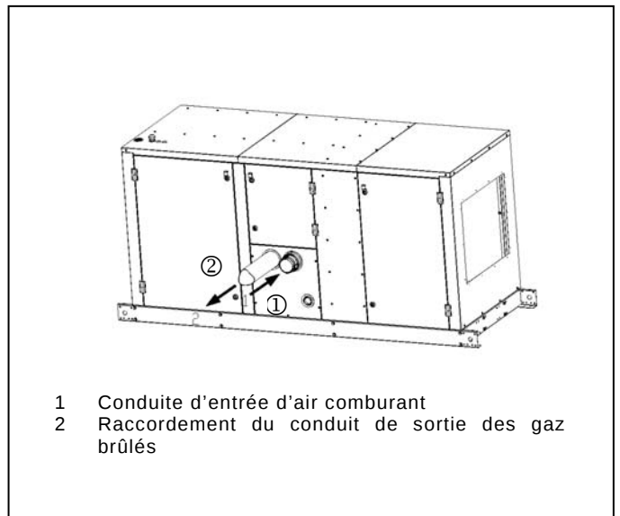
Figure 7b: Installation type B – raccordements conduits d'arrivée d'air comburant et d'évacuation des gaz brûlés
