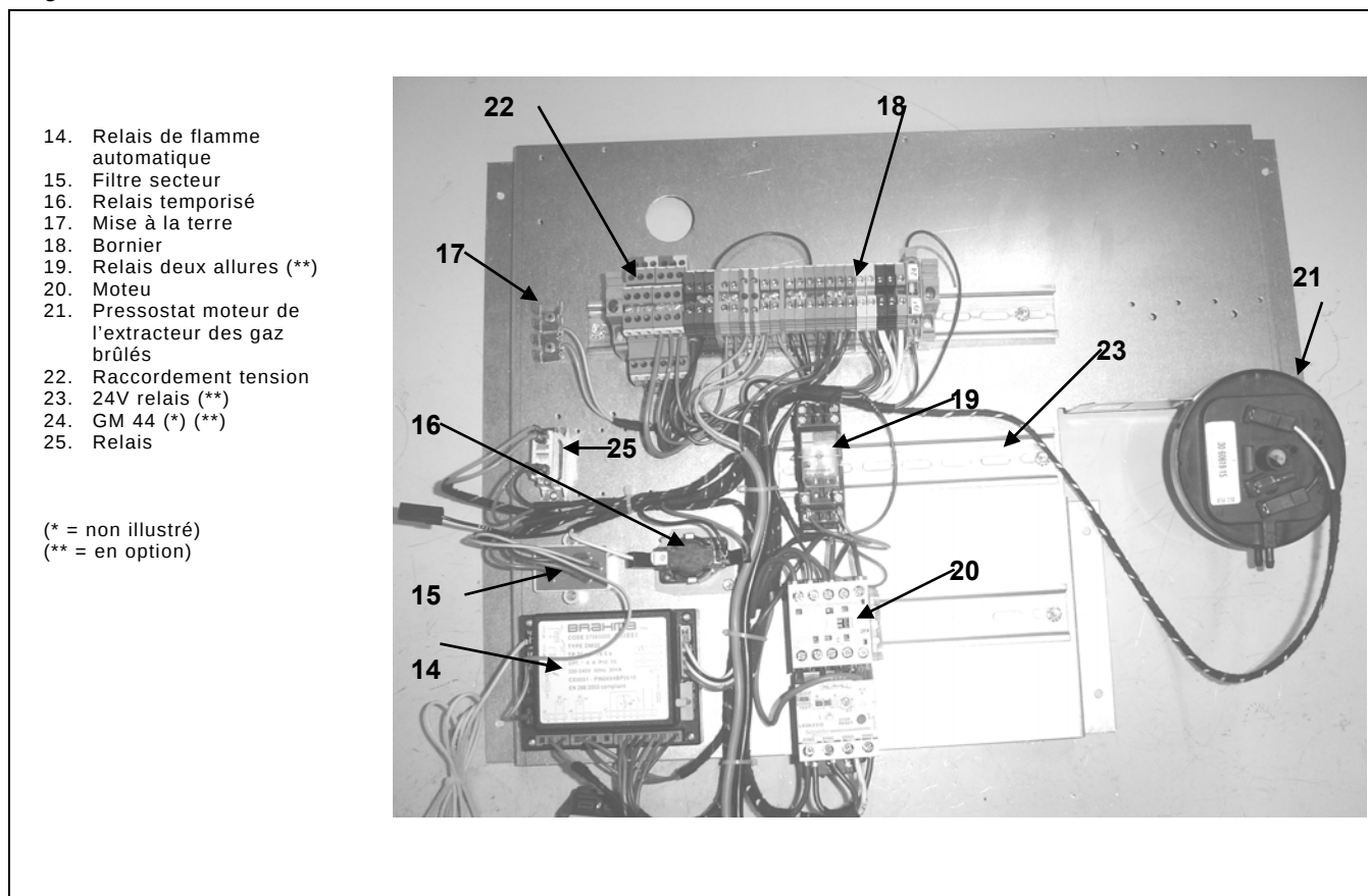
Figure 16b : Détail raccords au bornier
