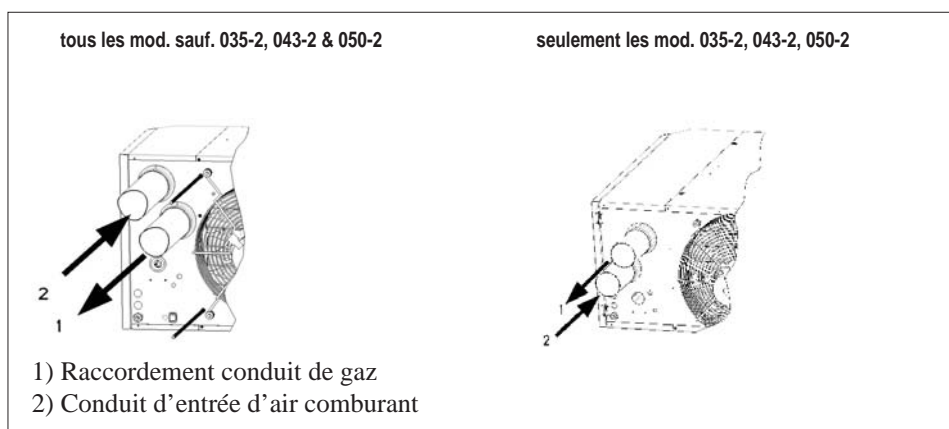
Figure 5 : Applications Type C : Raccordements conduits d'arrivée d'air comburant et d'évacuation des gaz brûlés
