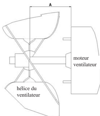
Figure 18 - Position des pales du ventilateur sur l'axe du moteur
