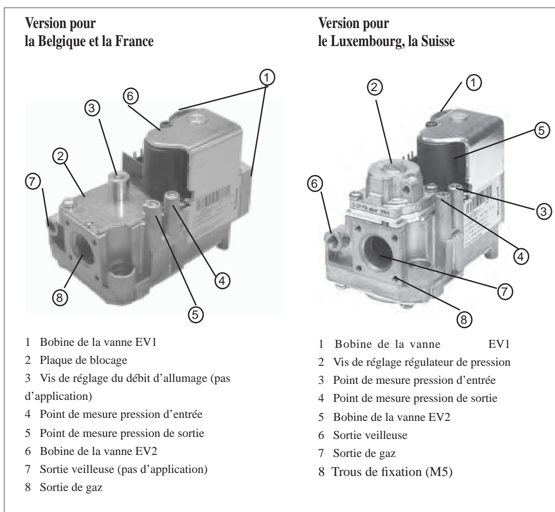
Figure 10a : Vanne de gaz HONEYWELL (types 008-2 >-032-2)
