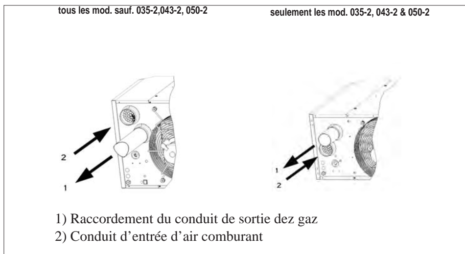
Figure 3 : Installation type B : Raccordements conduits d'arrivée d'air comburant et d'évacuation des gaz brûlés
