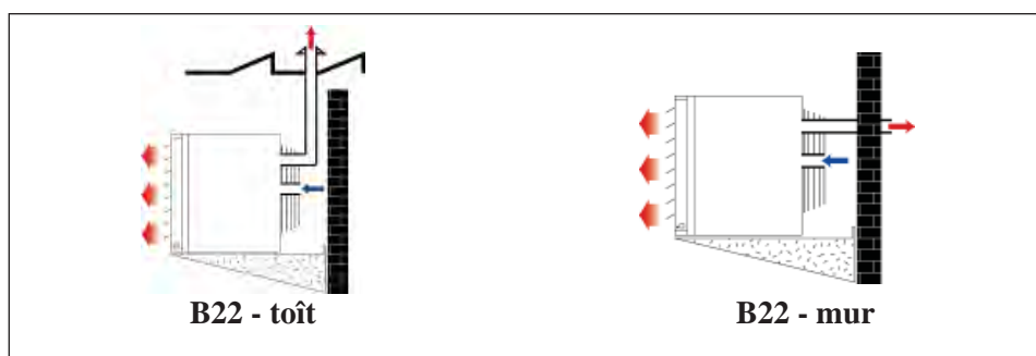
Figure 2 : Applications certifiées type B
