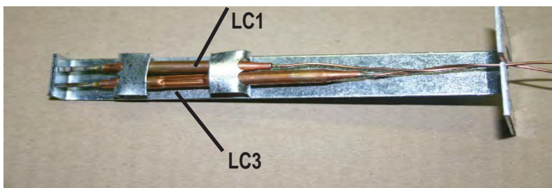
Figure 25 : Positionnement LC1/LC3
