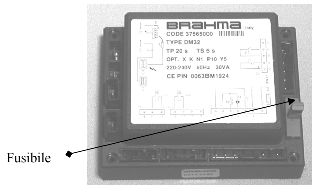
Figura 17 : Controllo bruciatore
